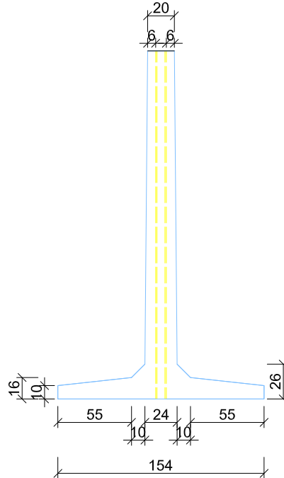
seccion A-A'
