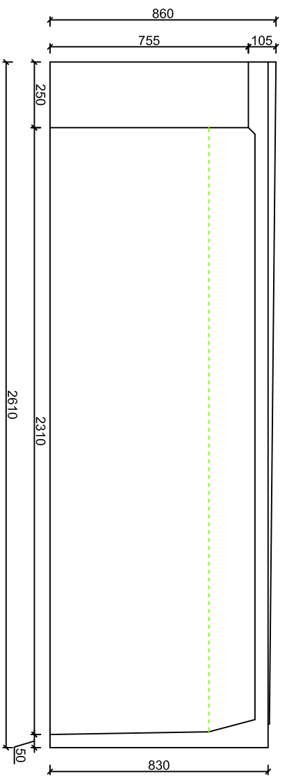
SECCION LONGITUDINAL
