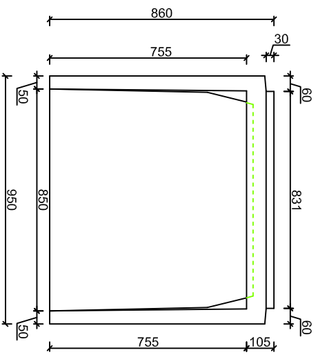
FRENTE-ALZADO
