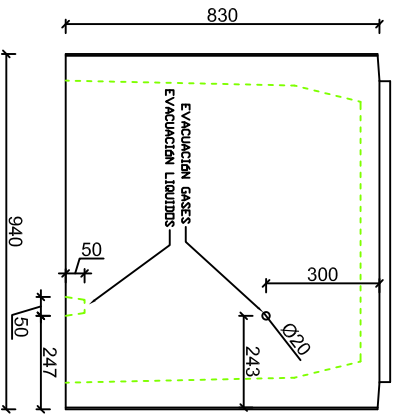
TRASERA-ALZADO
